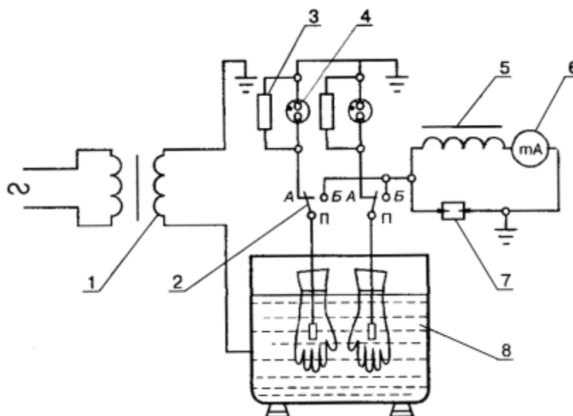
Рис. 2.4. Принципиальная схема испытания диэлектрических перчаток, бот и галош
