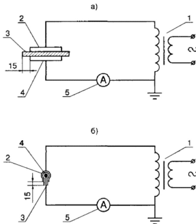
Рис. 2.6. Схемы электрических испытаний гибкого изолирующего покрытия (а) и гибкой изолирующей накладкой (б)
