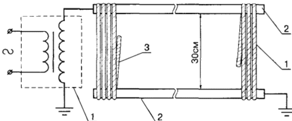
Рис. 2.5. Схема электрических испытаний изолирующего каната
