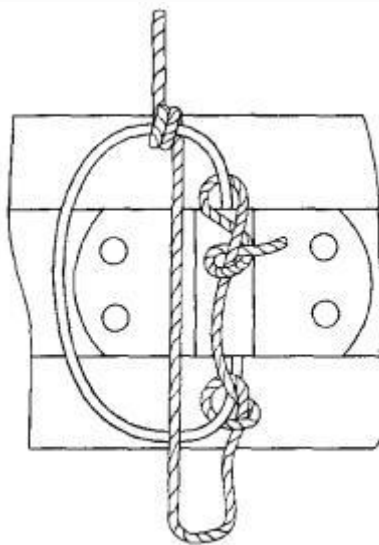
Рис. 2.7. Узел крепления страховочного каната к кольцу
