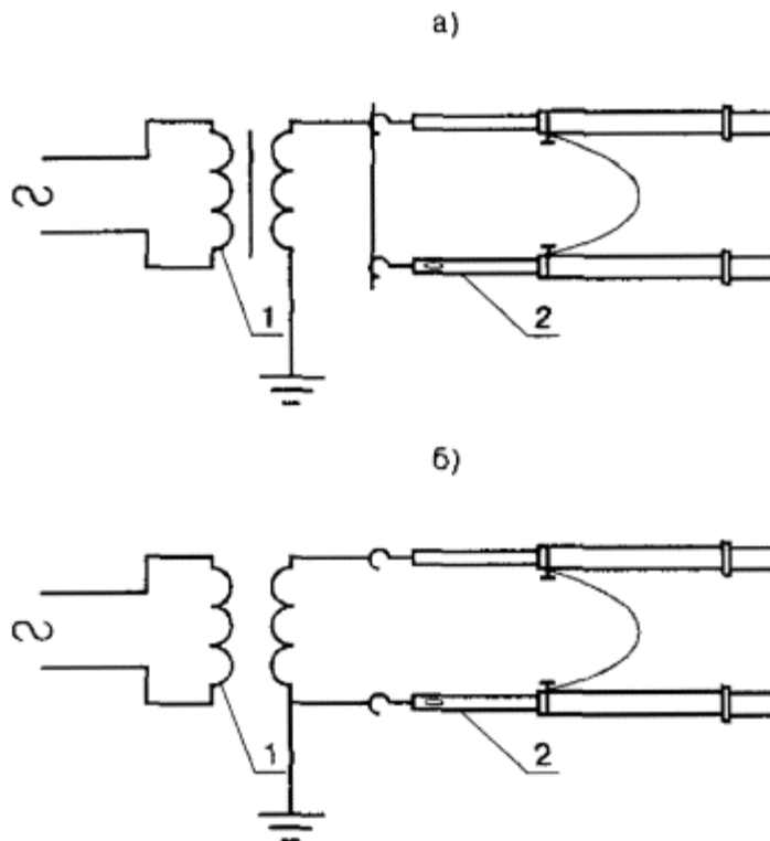
Рис. 2.2. Принципиальная схема испытания указателя напряжения для проверки совпадения фаз по схеме согласного (а) и встречного (б) включения:
